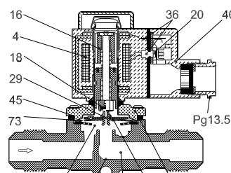
EVR 10 (NO)
