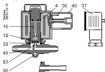
EVR 2 (NC)
