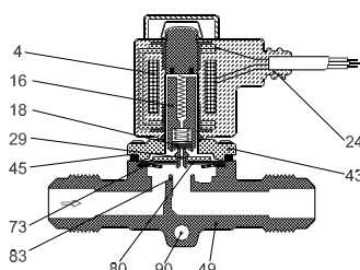
EVR 10 (NC)
