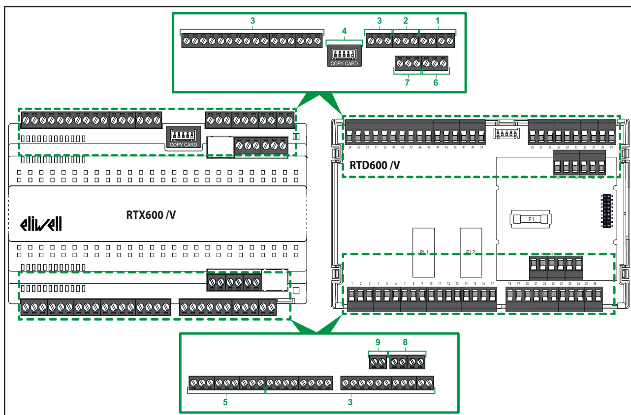
Рис. 4. Основные компоненты RTX-RTD 600 /V
