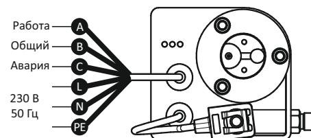
Рис.3. Электрические соединения
