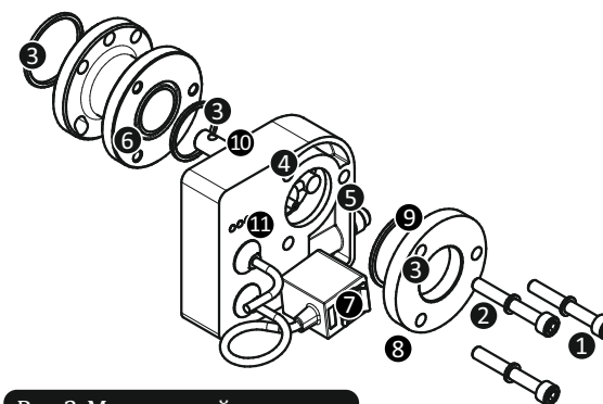
Рис.2. Монтажный чертеж
